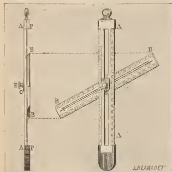
Fig. 3. - El similigrafo-nivel
